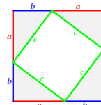
Pythagoras: vgl. Flächeninhalte
