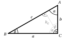
Rechtwinkeliges Dreieck
